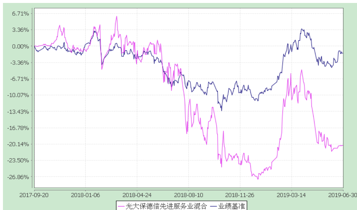
光大保德信先进服务业灵活配置混合型证券投资基金 份额累计净值增长率与业绩比较基准收益率历史走势对比图 (2017 年 9 月 20 日至 2019 年 6 月 30 日)
