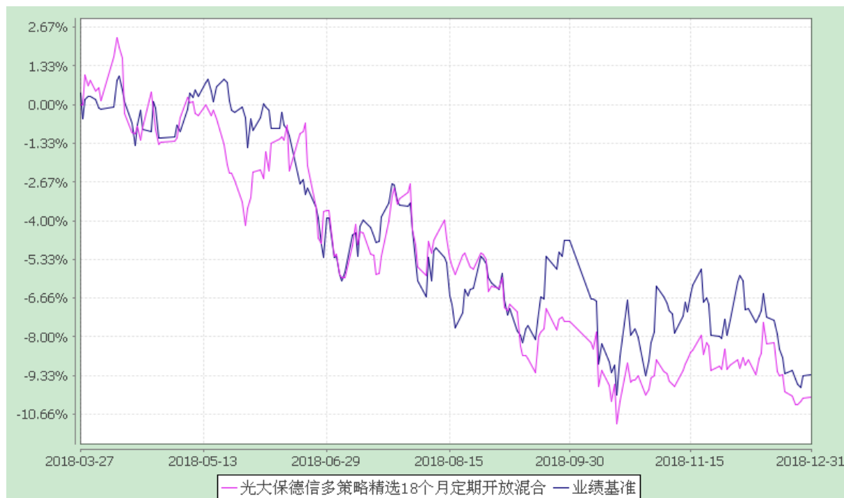
光大保德信多策略精选 18 个月定期开放灵活配置混合型证券投资基金 自基金合同生效以来份额累计净值增长率与业绩比较基准收益率的历史走势对比图 (2018 年 3 月 27 日至 2018 年 12 月 31 日)
